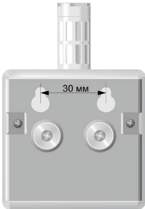
Рис.2 – Универсальное крепление на обратной стороне прибора
